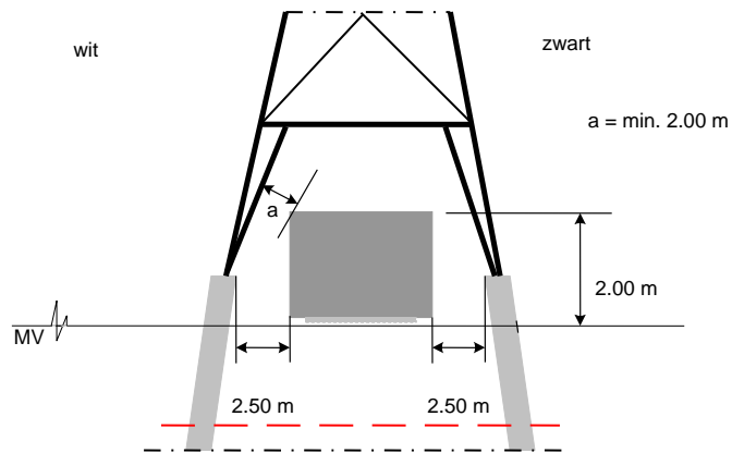
zijaanzicht stapaarde en plaats apparaatruimte/ hekwerk tussen mastpoten
